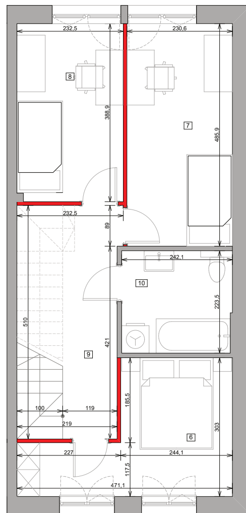
PIĘTRO
